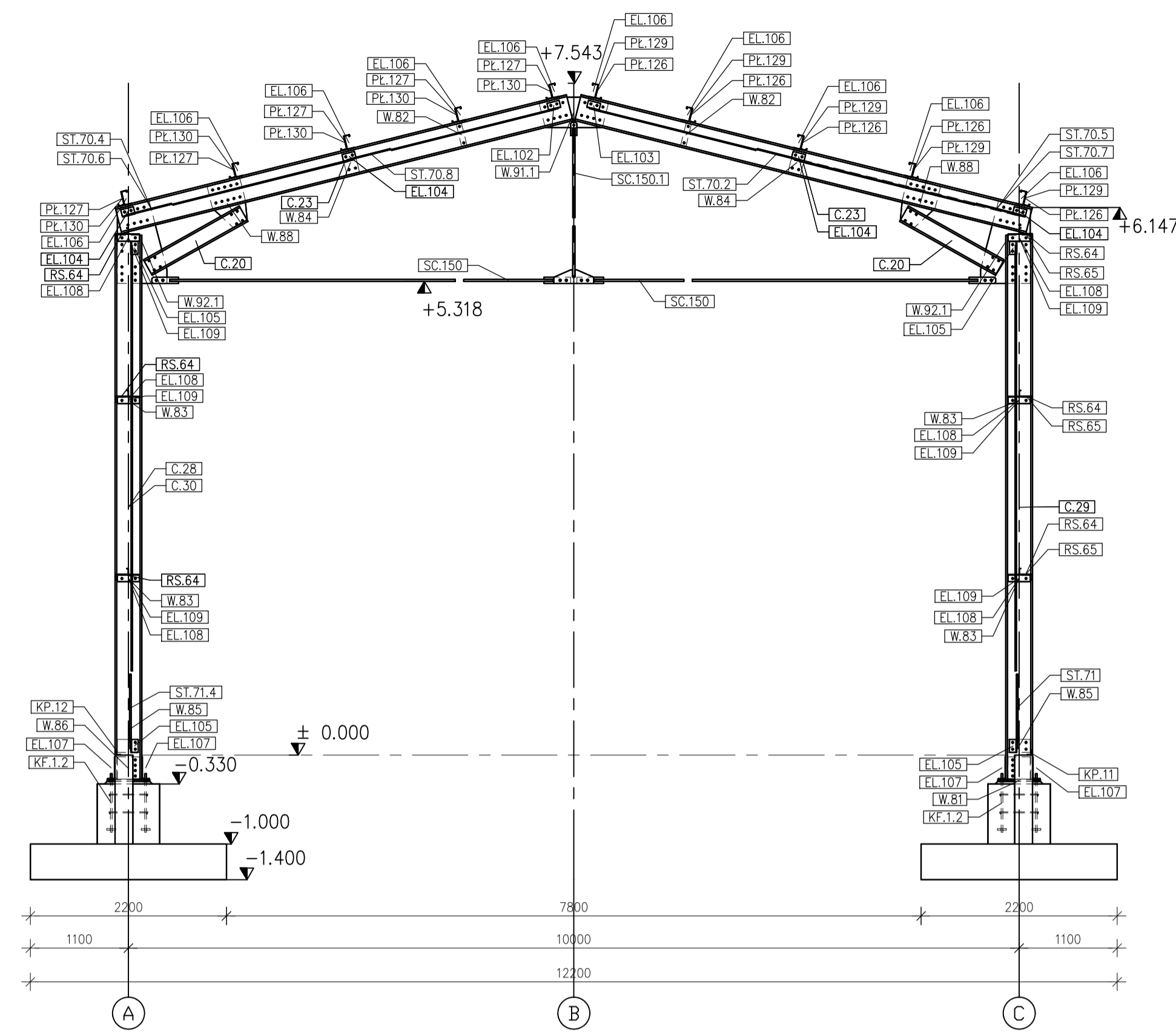
Przekrój w osi "2" (Sc1:50)
