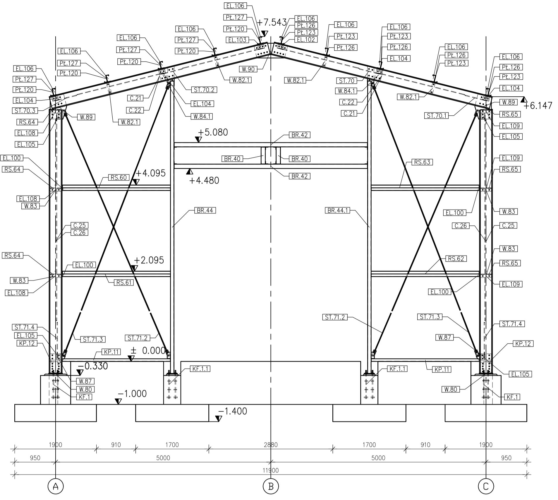
Przekrój w osi "1" (Sc1:50)
