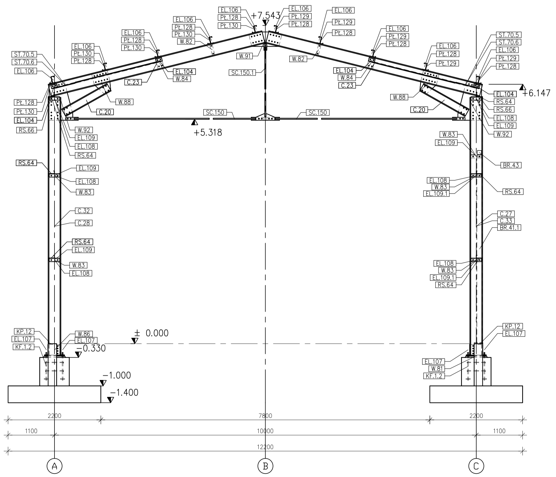
Przekrój w osi "3" (Sc1:50)
