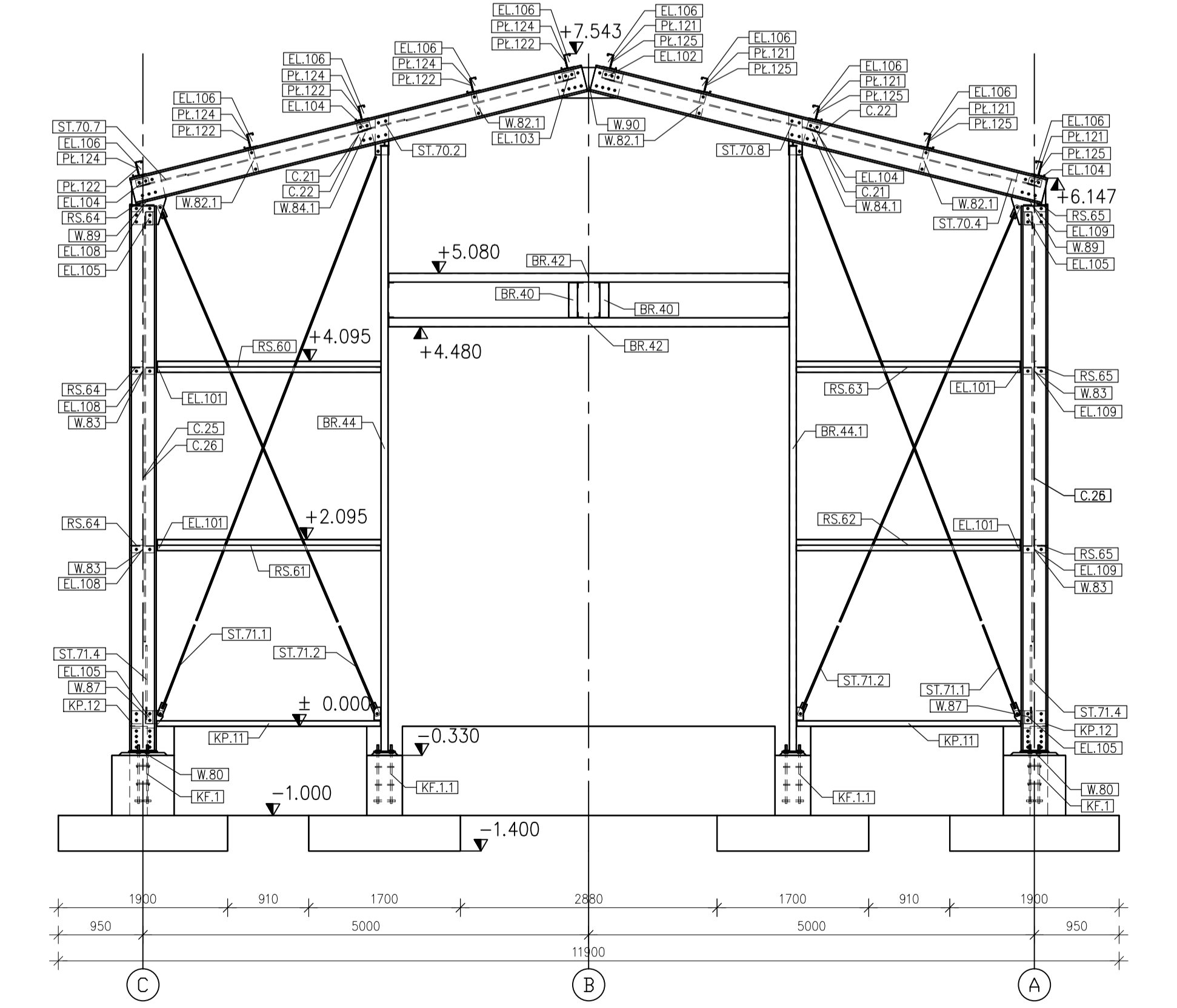
Przekrój w osi "9" (Sc1:50)
